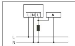
Bei Schaltung von Induktivitäten (z. B. Relais, Schütze, Vorschaltgeräte) kann der Einsatz eines Löschlides (A) erforderlich sein.
